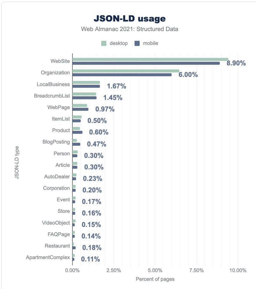
Figure 4.10. JSON-LD usage
