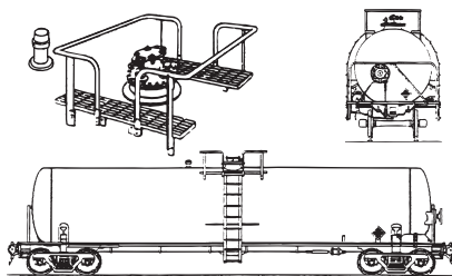
Carrotanque de baja presión para líquidos (Domo Cerrado y Válvulas en la Parte Superior)
