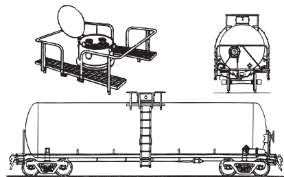
Carrotanque presurizado para gases licuados comprimidos (Domo Cerrado sólo en la Parte Superior)
