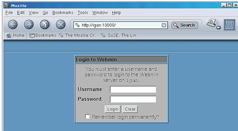
Figure 4-7 Webmin login
